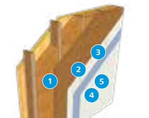
...og STEICOjoist
