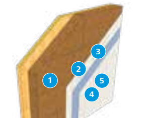
Med massiv trævæg
