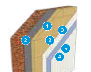
Med klæbemørtel c)
