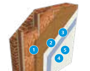
Teglvæg med STEICOjoist
